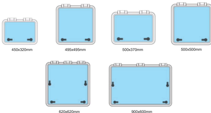
Standard Luke mit 5 mm tiefem Flansch (senkrechte Nase nach unten)
