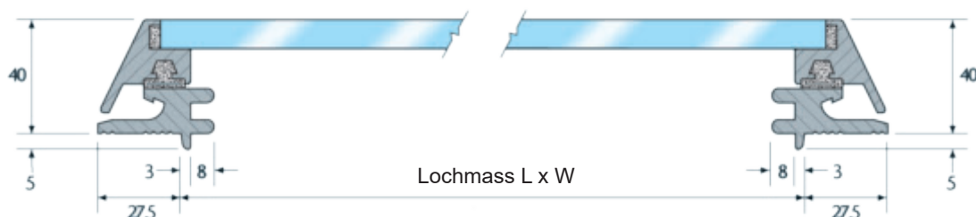
Standard Luke mit 5 mm tiefem Flansch (senkrechte Nase nach unten)
